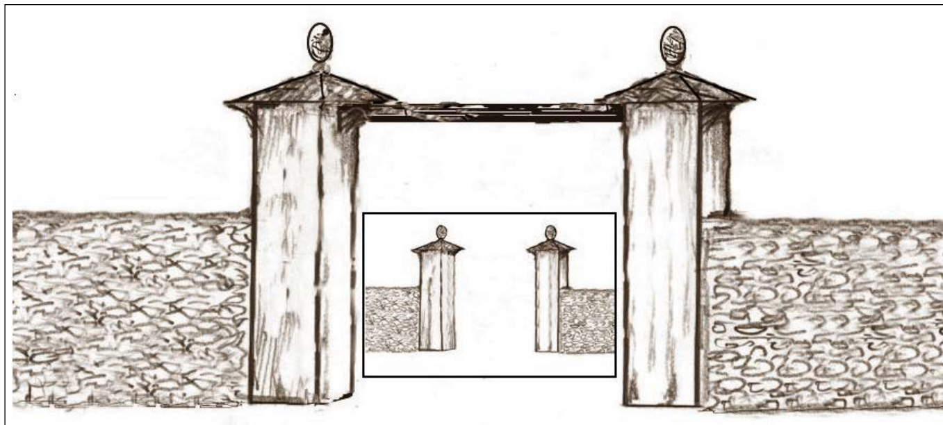
Obr. Rozpěrné trámové nadpraží Vyškovské brány v 18. a 19. století a pohled bez nadpraží.
